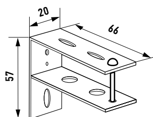
Установочный кронштейн 245780
