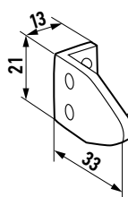
Держатель карниза для нижней фиксации 240175-0000
