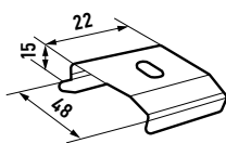
Кронштейн потолочный
